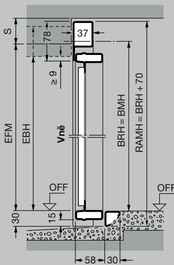
Svislý řez Vrata se spodním dorazem
